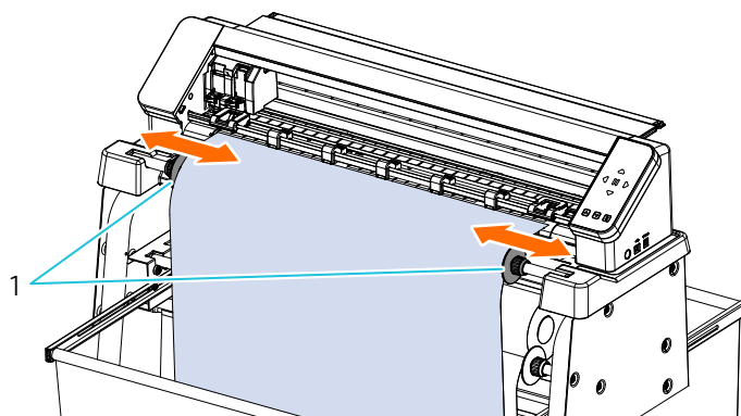
1. Flanges
